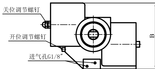
QZ8~20外形尺寸图
